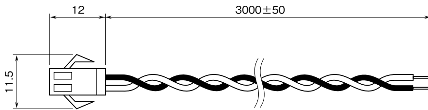
外形寸法図 (単位: mm)
