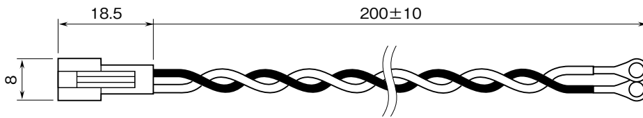
外形寸法図 (単位: mm)
