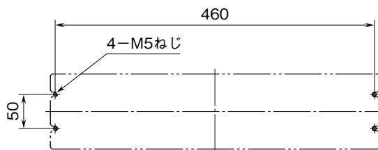
取付寸法図 (単位: mm)
