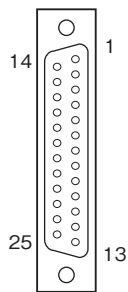
■コネクタピン配列
