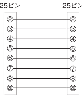
■配線図
