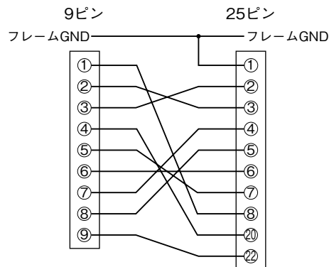
■配線図
