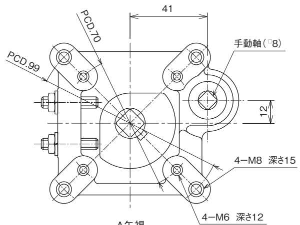
A矢視
