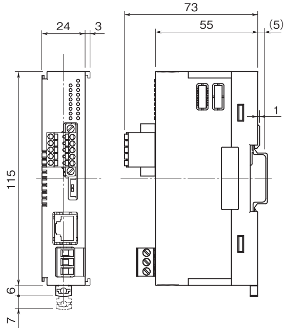
■単独設置形
