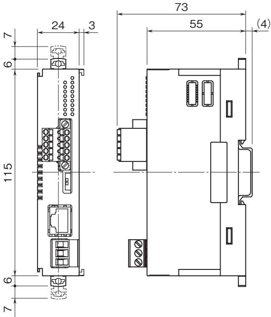
■DL8連結形
