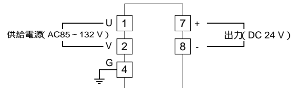
端子接続図
