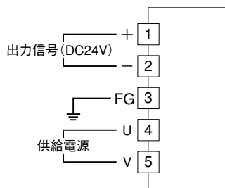
端子接続図
