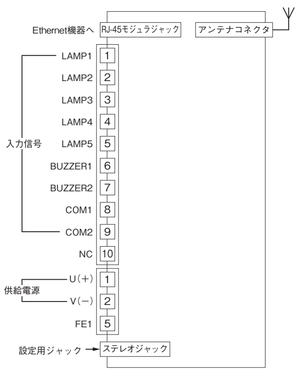
■入力信号との配線 ・接点入力接続例
