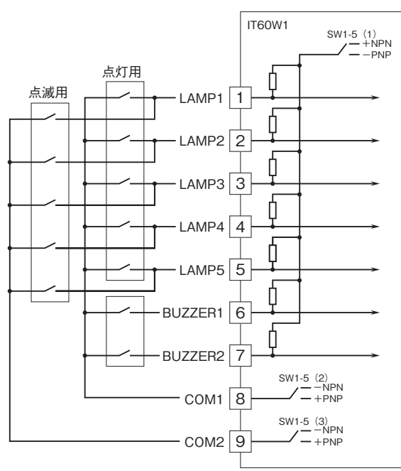
■入力信号との配線 ・接点入力接続例
