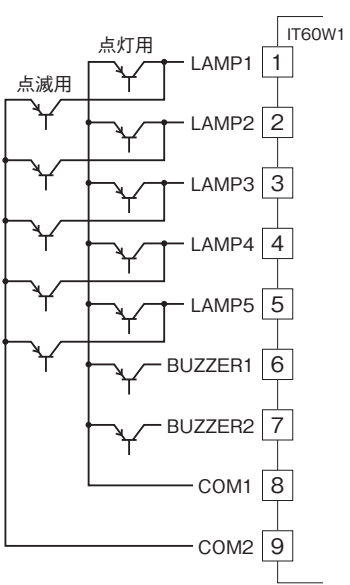
・ PNP入力例
