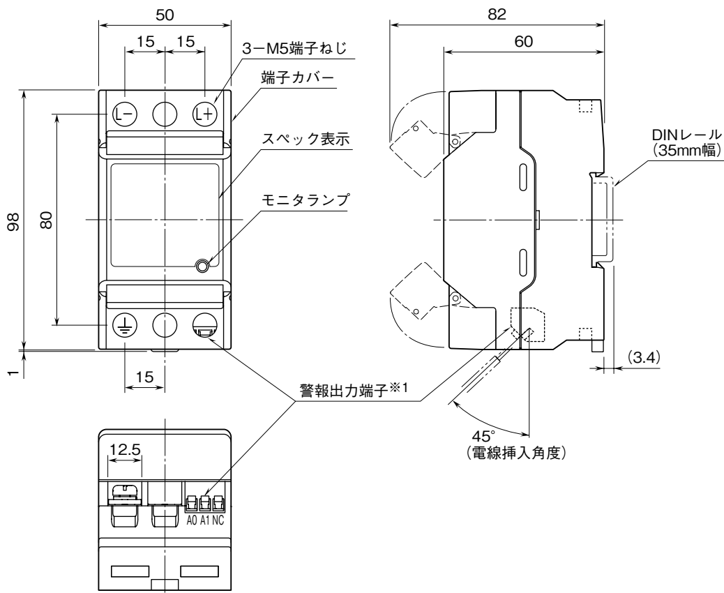
外形寸法図 (単位: mm)
