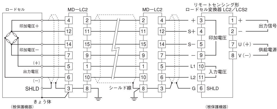
端子接続図
