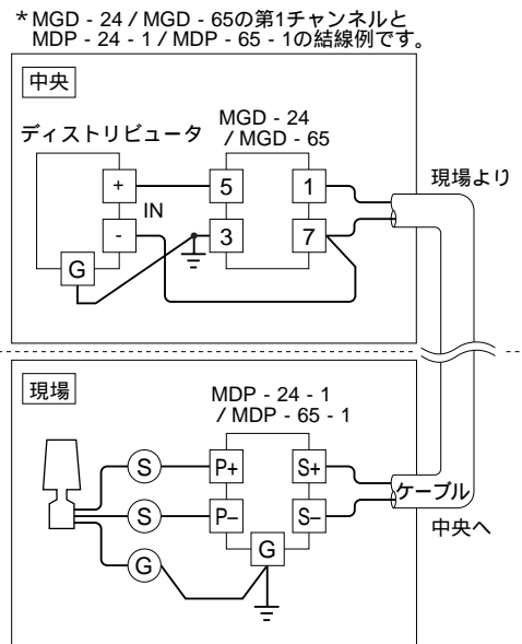
端子接続図
