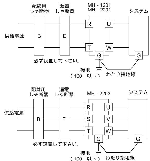
端子接続図
