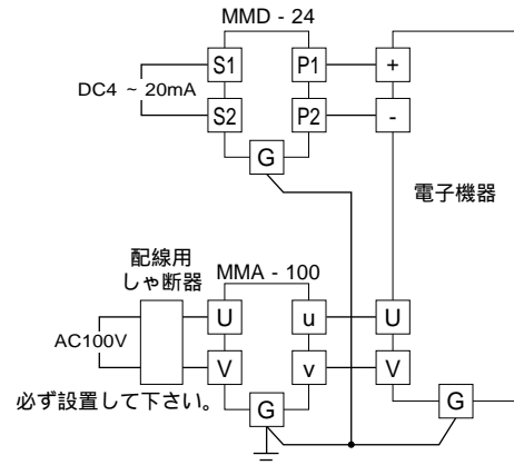
端子接続図
