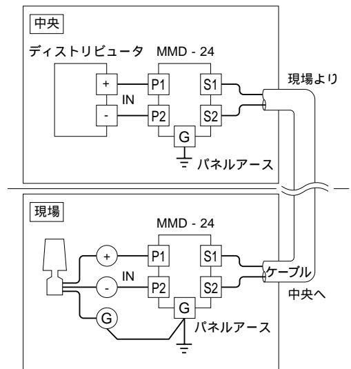
端子接続図
