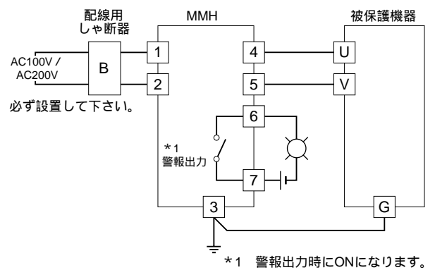
端子接続図
