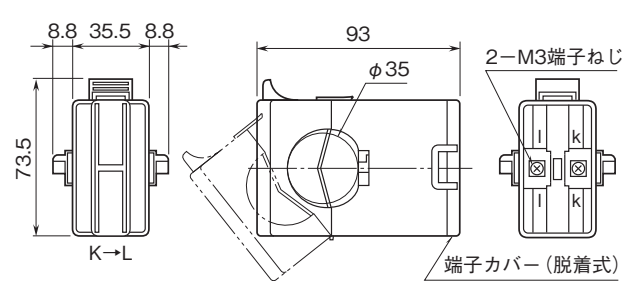
■クランプ式センサ:CLSB-40
