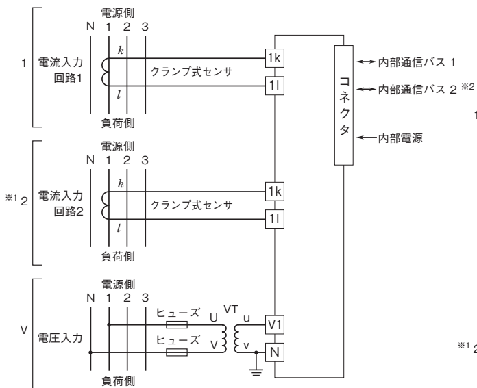
■三相4線 平衡負荷
