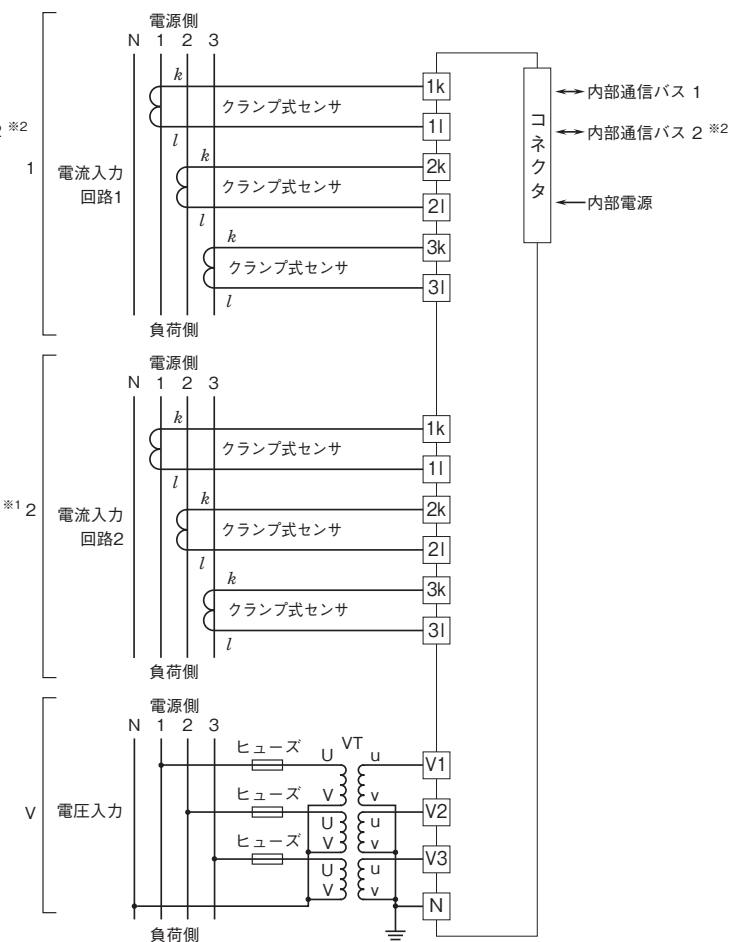
■三相4線 不平衡負荷3線
