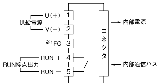
端子接続図
