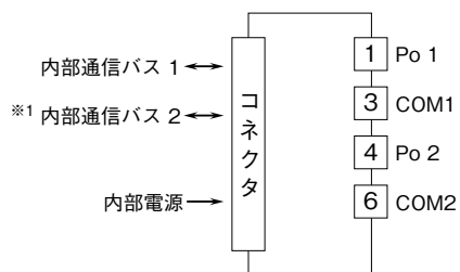
端子接続図
