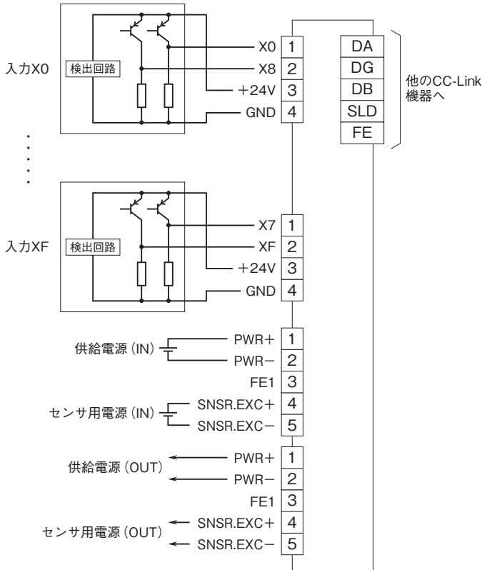
■2線式センサの場合
