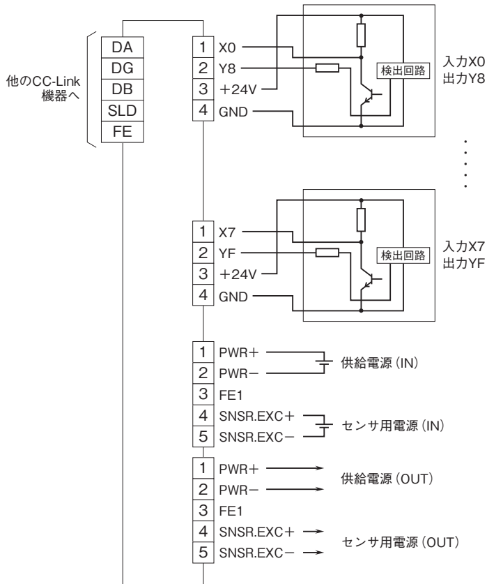
■2線式センサの場合
