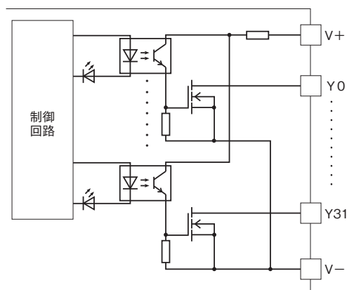
■出力回路
