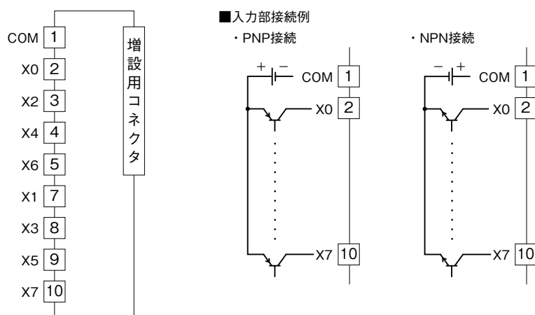
端子接続図
