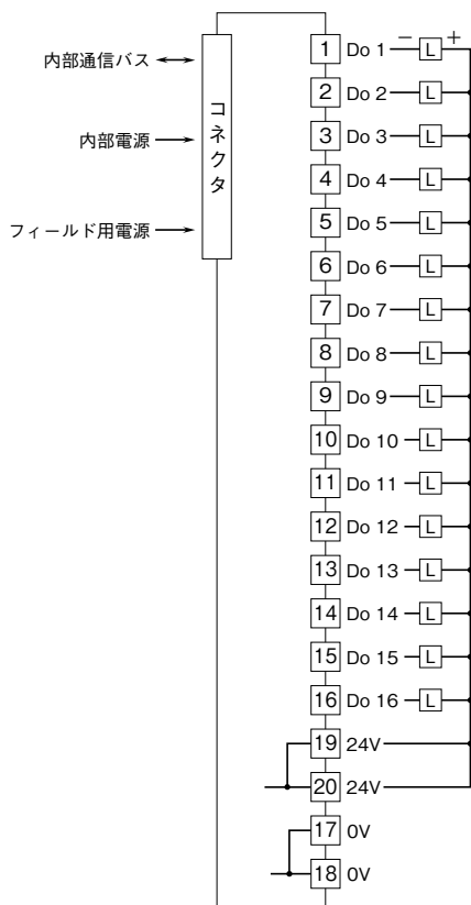
端子接続図
