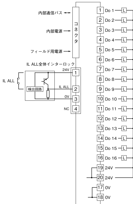
端子接続図
