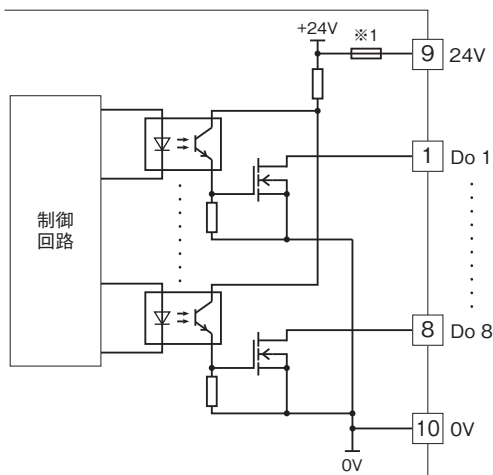
■出力回路
