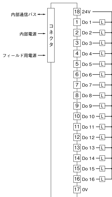
端子接続図
