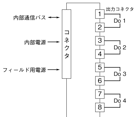
端子接続図
