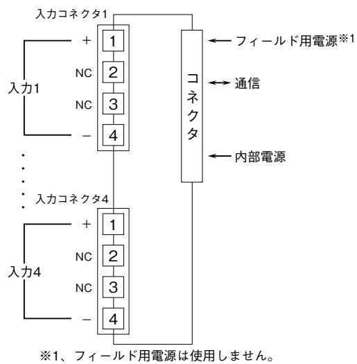
端子接続図
