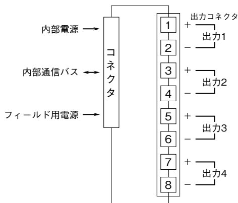
端子接続図
