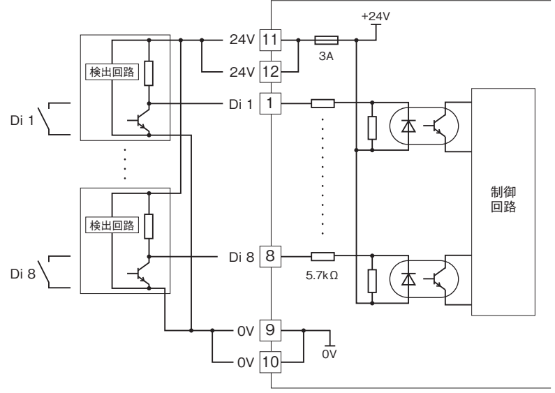
■入力回路
