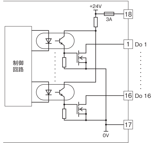
■出力回路
