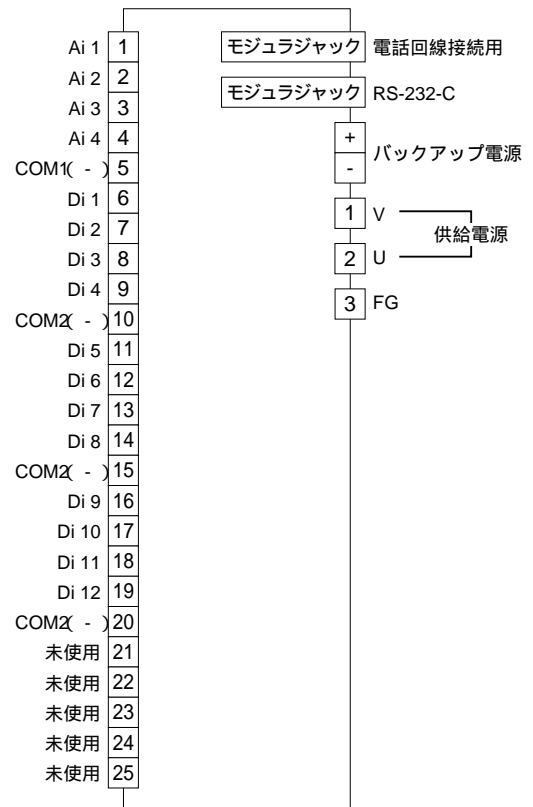
端子接続図
