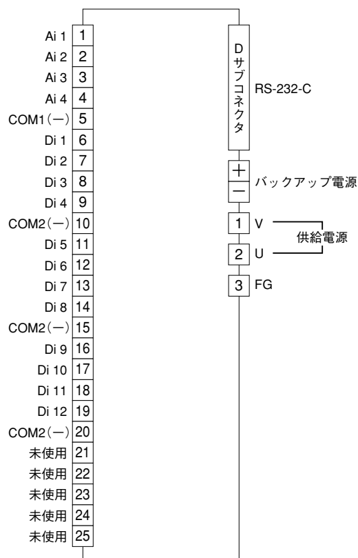
端子接続図
