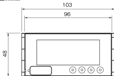
■前面図
