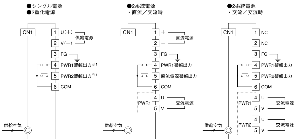
端子接続図
