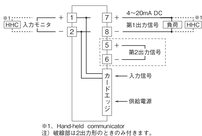
端子接続図
