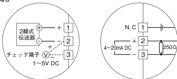
図A フィールド用端子接続図
