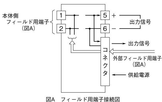
図A フィールド用端子接続図
