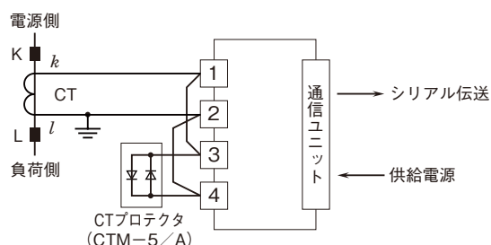
端子接続図
