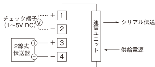
端子接続図
