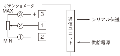
端子接続図
