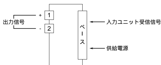
端子接続図
