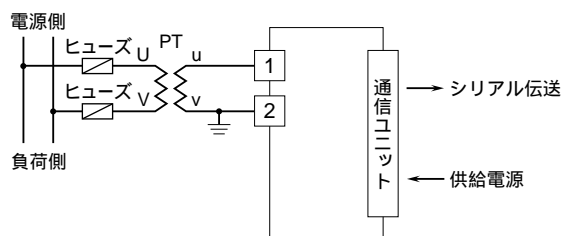
端子接続図
