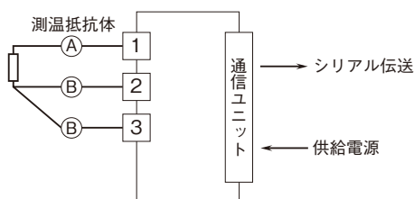
端子接続図
