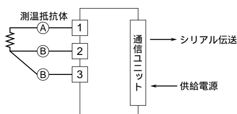
端子接続図
