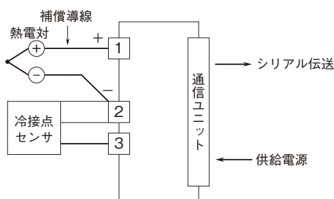
端子接続図
