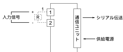
端子接続図
